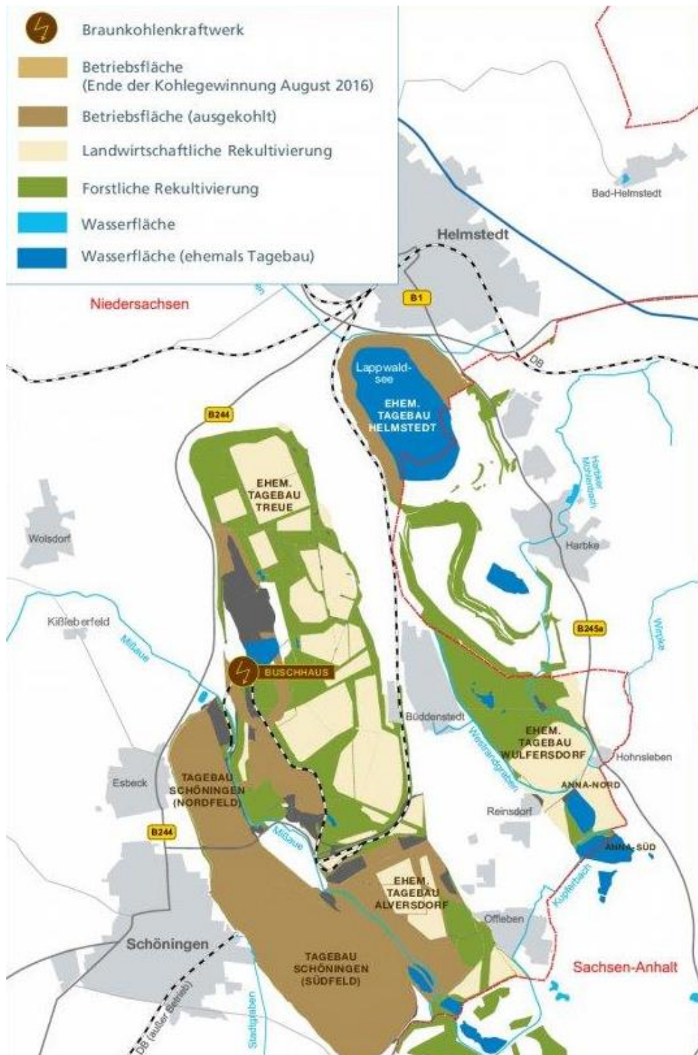
Abbildung 22, Helmstedter Revier (Quelle: DEBRIV 112 )
